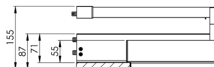
Tiroir avec rail - Vue profil
