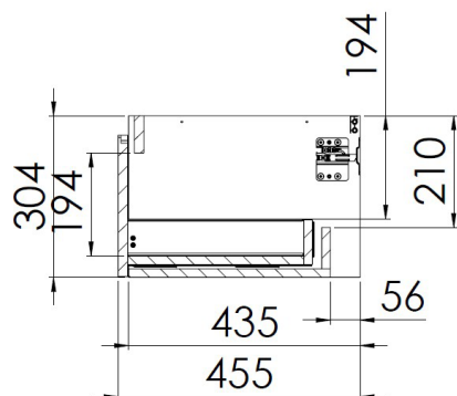
Tiroir simple - Vue profil
