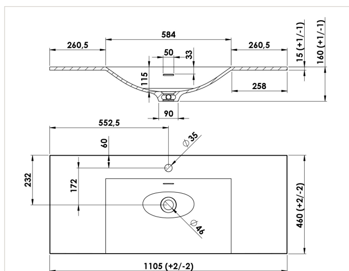
TEPLANC110... centré
