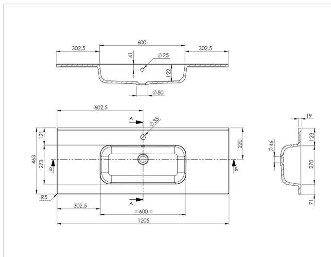
PRPLANC120BLB centré
