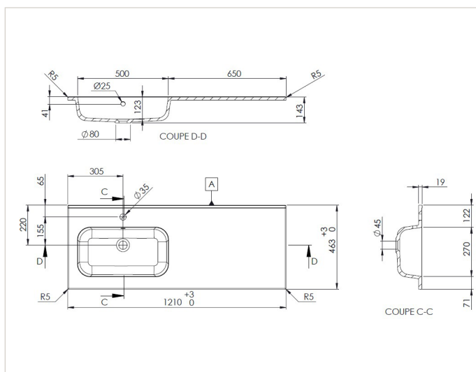
PRPLANG120BLB gauche
