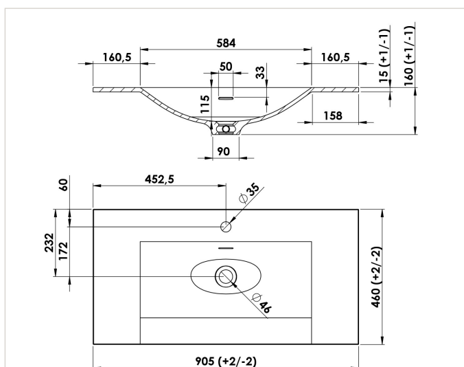
TEPLANC90...
