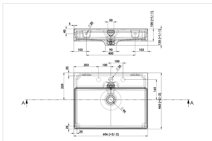
OGPLANC060...
