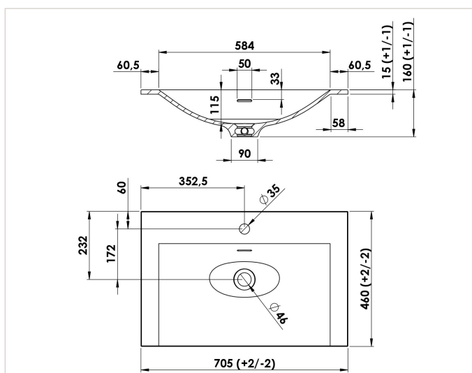
TEPLANC70...
