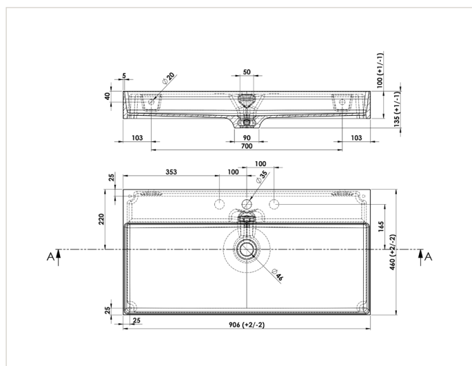
OGPLANC090...
