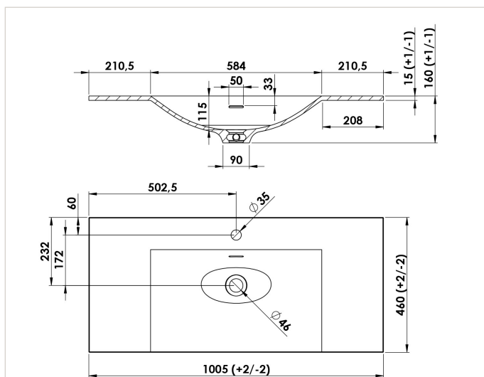
TEPLANC100... centré
