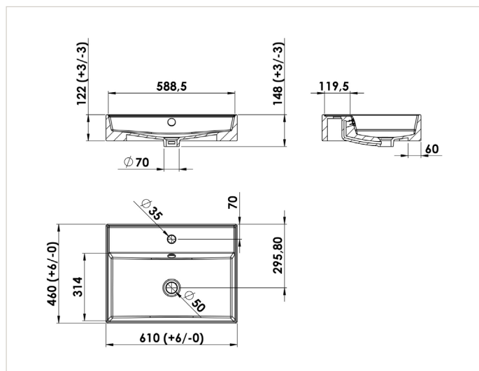
SEPLANC060CERB
