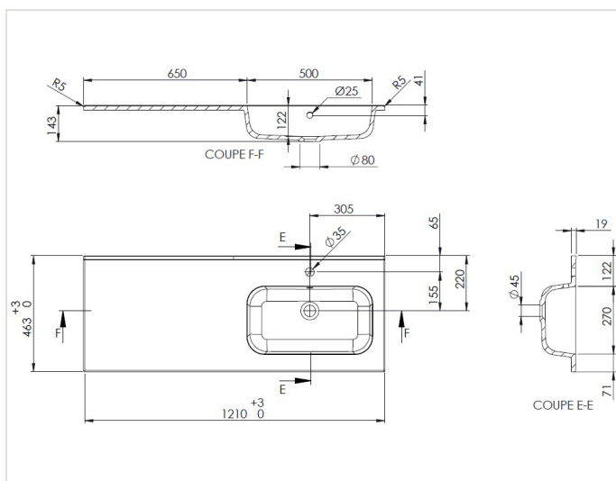
PRPLAND120BLB droite
