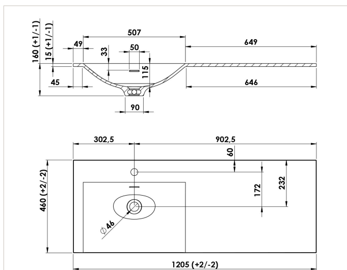
TEPLANG120... gauche
