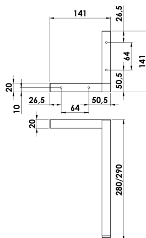
uniquement pour plateau + bol (pour avoir une hauteur de pose finale du bol de 87 à 94 cm par rapport au sol) Tube 20x20 mm. Patins de réglage de 10 mm.
