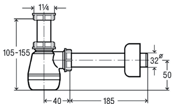
Siphon recoupable
