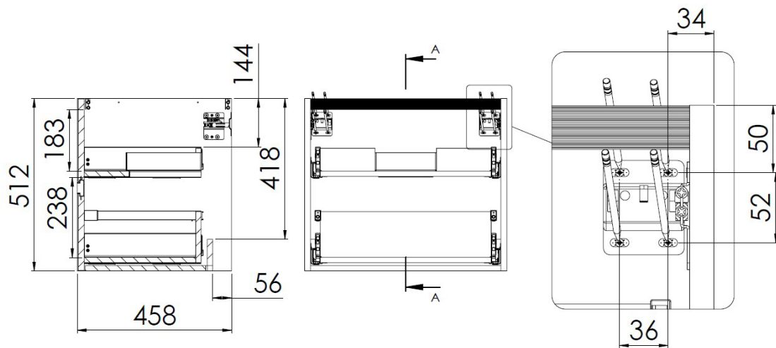
Tiroir simple - Vue profil
