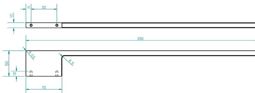
A fixer sur le côté du meuble. Perçage à effectuer sur chantier.
