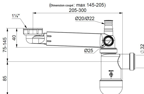
Siphon recoupable et extensible
