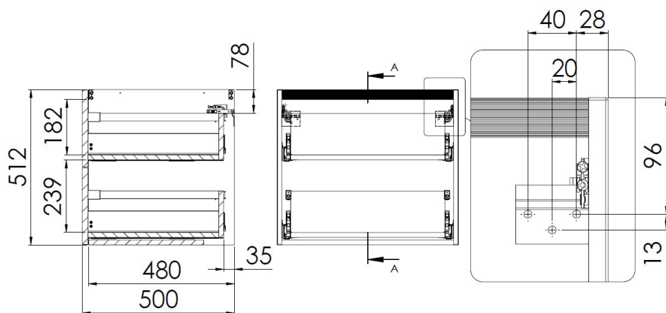
Tiroir simple - Vue profil
