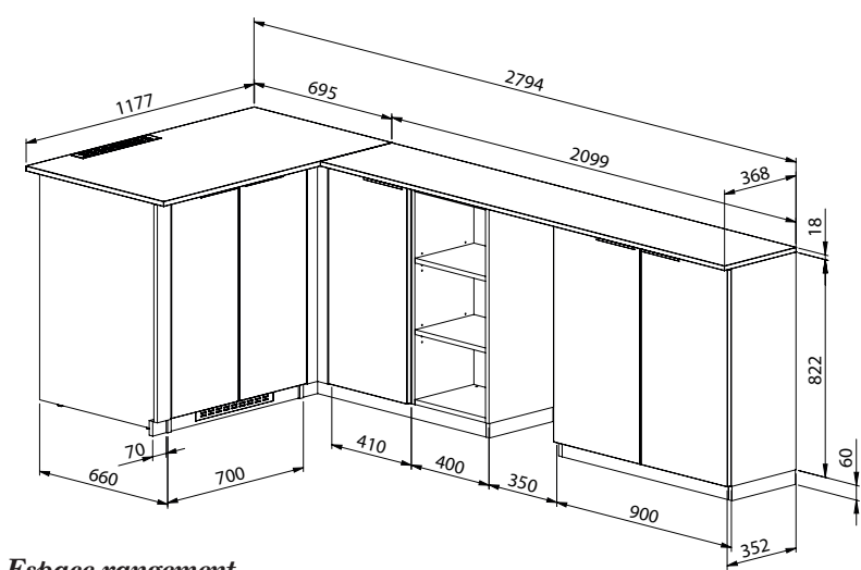
Aménagement hauteur 82 cm, profondeur 35 cm (disponible également en profondeur 45 et 58 cm)
