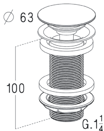
En laiton chromé brillant - pour utilisation avec vasque sans trop-plein incompatible mitigeur à tirette
